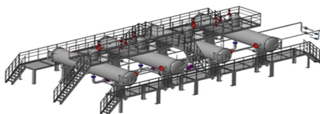
Блок очистки воды производительностью до 10 000 м 3 /сут
