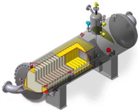
Блок очистки воды (в разрезе)
