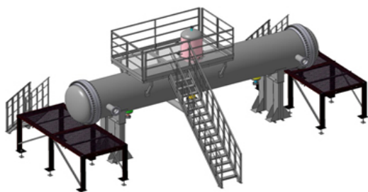
Блок очистки воды производительностью до 3000 м 3 /сут
